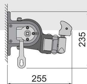
Montaż do ściany
