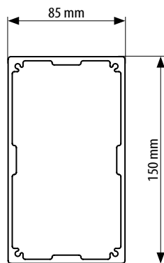
przekrój profilu konstrukcyjnego
