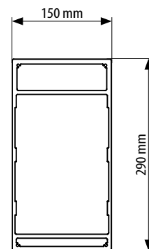
przekrój belki
