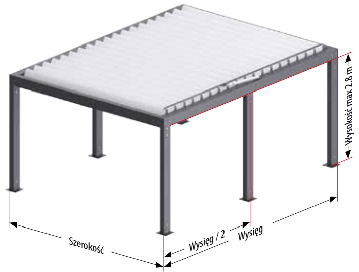
Wersja II dla pergoli o wysięgu powyżej 5.2 m posiada słup pośredni wspierający konstrukcję.
